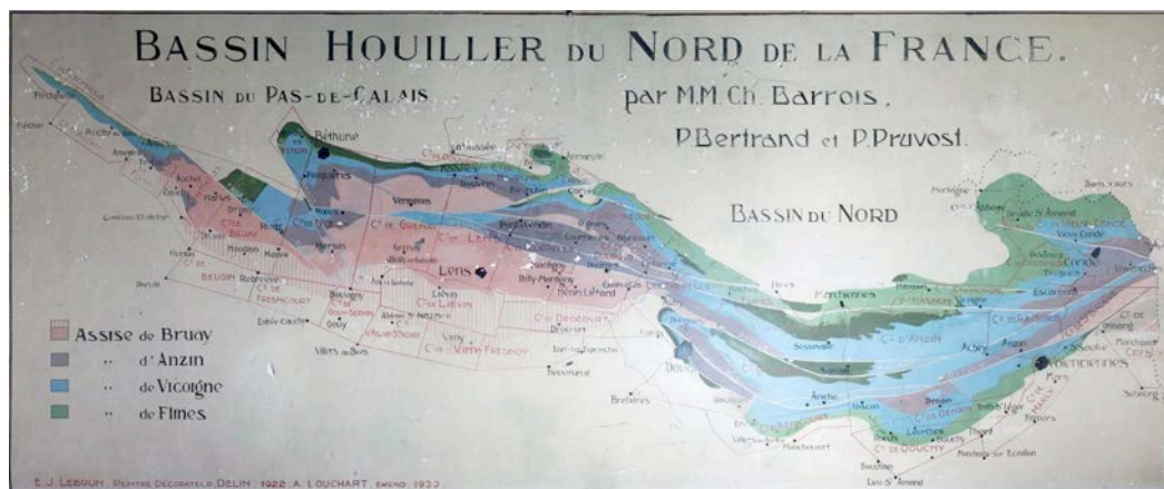
Carte géologique murale du bassin houiller du Nord – Pas-de-Calais (d'après Meilliez et al. 2014, Mémoire SGN n° XVII, Pl. II : 3)
